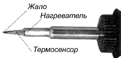
Рис. 1. Близость сенсора к точке пайки — залог точности измерения температуры
