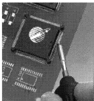
Рис. 3. Групповая пайка выводов жалом MicroWell
