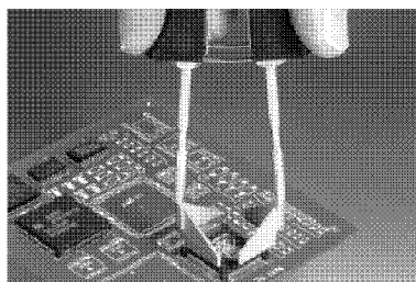
Рис. 4. Демонтаж SMD компонентов при помощи термопинцета
