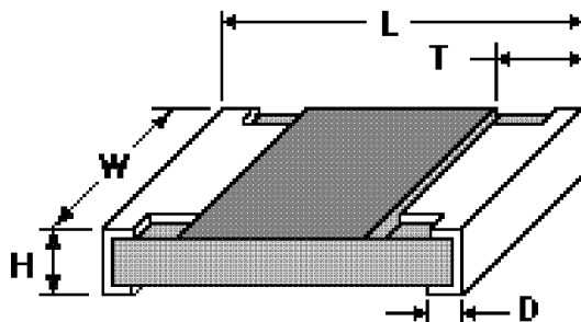
Рис. 1. Внешний вид чип-резистора
