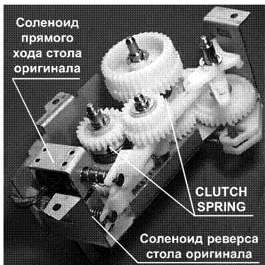
Рис. 3. Блок привода стола оригинала для RX 5009
