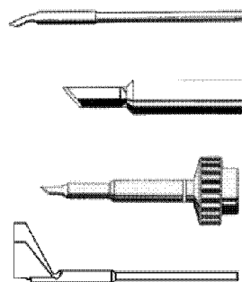
Рис. 2. Разновидности конструкции паяльных жал
