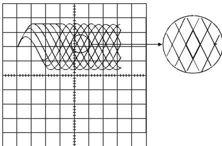
Рис. 3. Требуемый вид осциллограммы при проверке CD-проигрывателя
